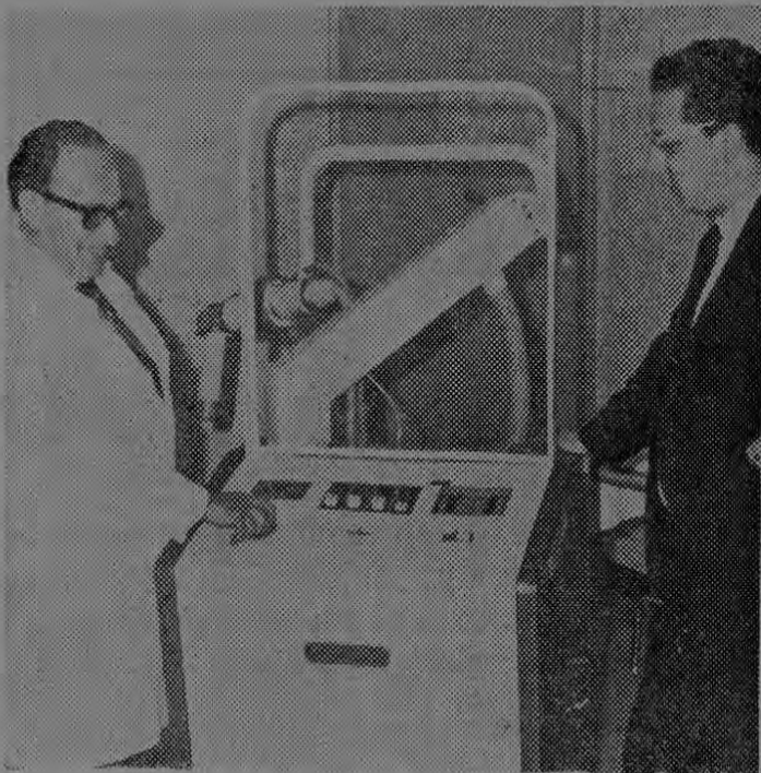
RADIACION SUPERFICIAL. — El tratamiento del cáncer es distinto según el tipo, su ubicación y su modalidad. El Dr. Núñez explica al periodista Carlos Mora de LA PRENSA LIBRE la forma en que funciona el aparato para aplicar radiación superficial.
