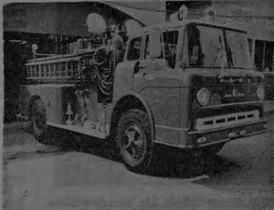
Moderna máquina para apagar incendios, destacada por el INS en Limón, Cuenta con compartimientos especiales de Bióxido de Carbono y Espuma, agentes especiales para combatir incendios en refinerías de petróleo.
